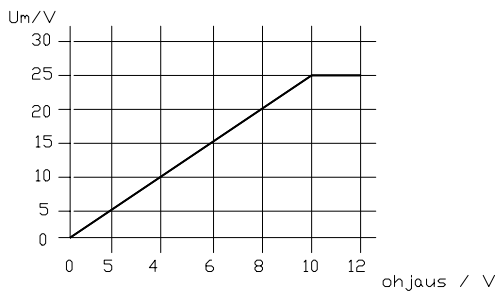
ohjausjännite / moottorijännite
